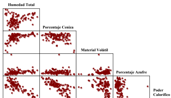
Fig. 4. Matriz de correlación de las propiedades del carbón medidas en la pila de almacenamiento.
