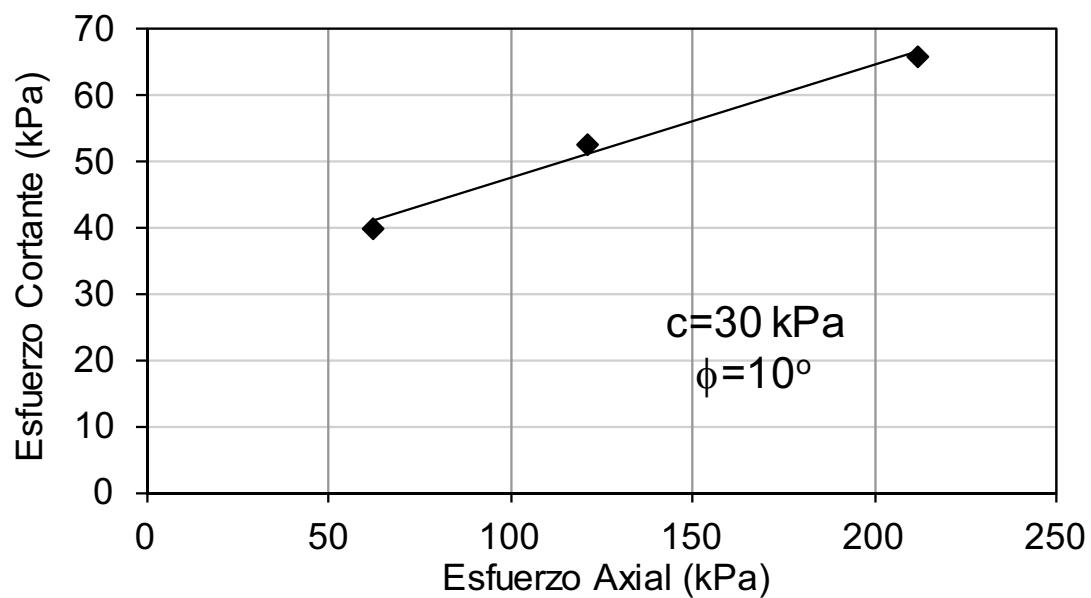
Fig. 5. Resultados ensayo de corte directo Fuente: Elaboración propia
