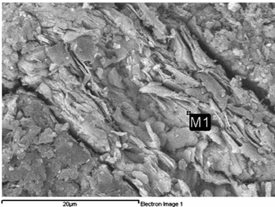
Fig. 4. Microscopía electrónica de barrido Fuente: Elaboración propia
