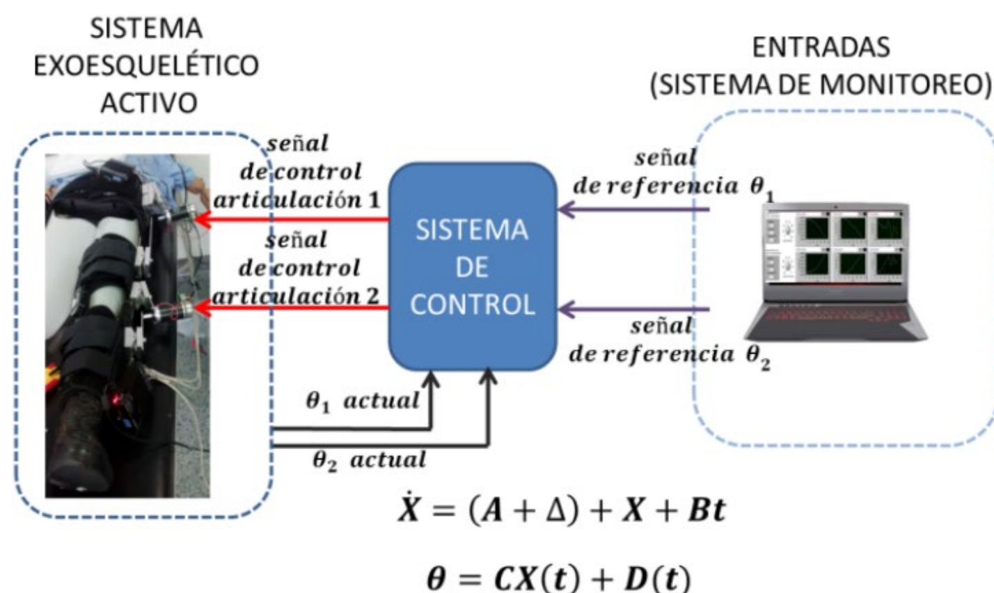
Fig. 6. Sistema de control
