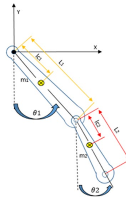
Fig. 4. Descripción del sistema de dos eslabones Fuente: Autores.
