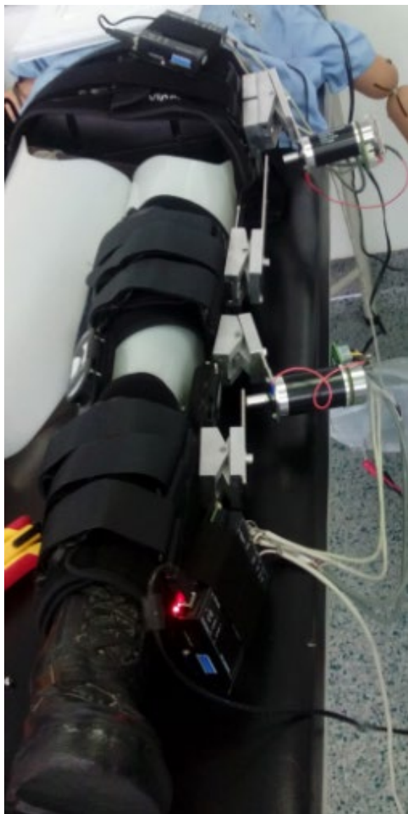
Fig. 9. Exoesqueleto desarrollado y plataforma para pruebas.
