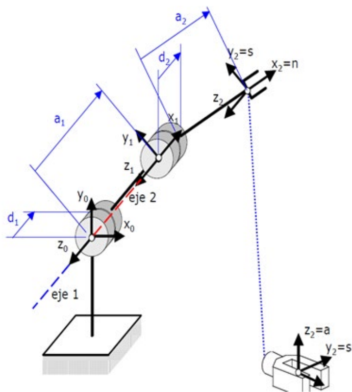
Fig. 3. Sistema de coordenadas en miembro inferior Fuente: Autores.
