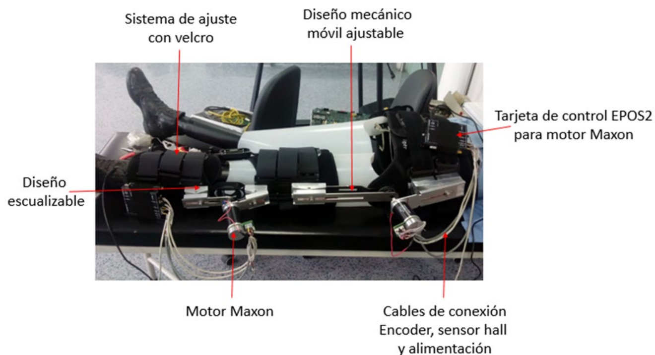
Fig. 8. Exoesqueleto desarrollado.
