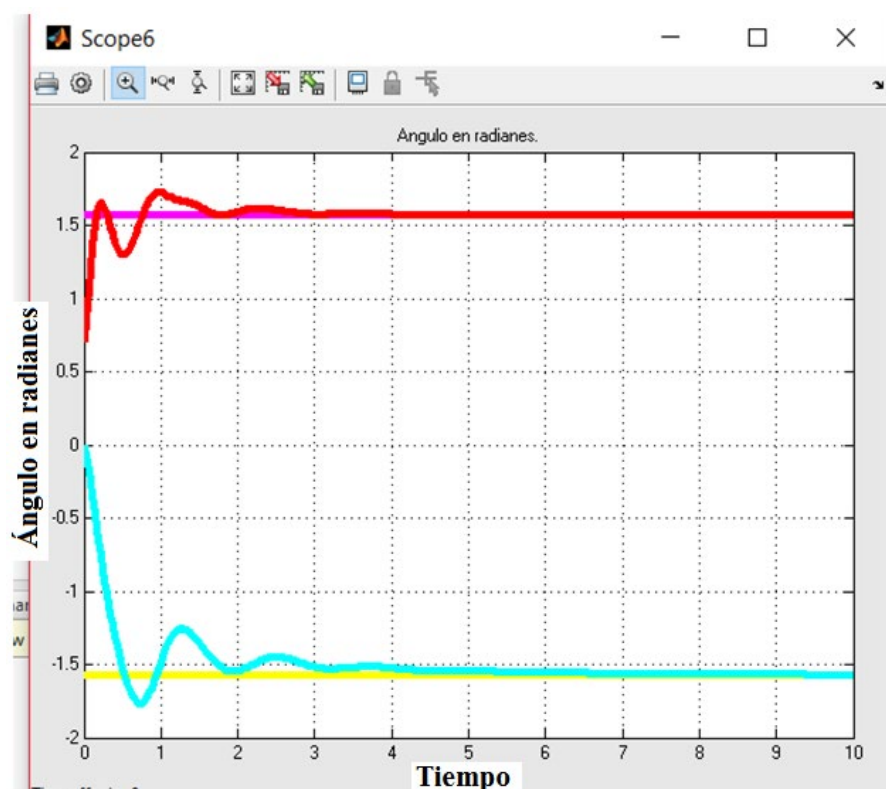
Fig. 7. Respuesta del controlador PID con realimentación de velocidad diseñado.
