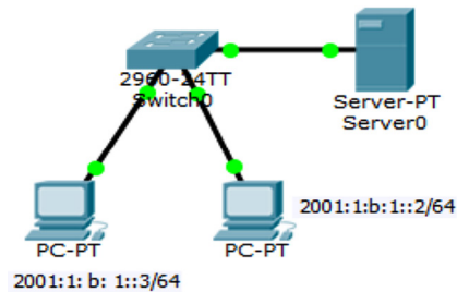
Fig. 10. Escenario para SSH bajo IPv6. Fuente: Autor.
