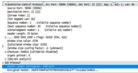
Fig. 12. Mensaje encriptado entre extremos con IPv6. Fuente: Autor.
