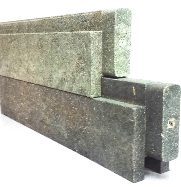
Figura 8. Ladrillo realizado con plástico reciclado Fuente: https://ecoinventos.com/casas-de-ladrillos-de-plastico/
