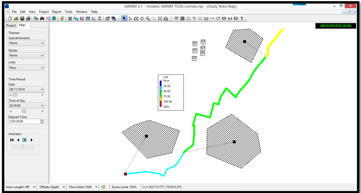
Figura 73. Representación de los caudales para un periodo de retorno T_r=50 años
