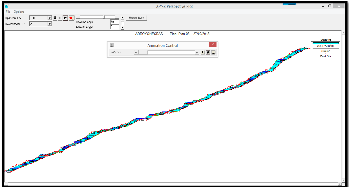
Figura 76. Perfil correspondiente para un periodo de retorno de 2 años obtenido en HEC-RAS
