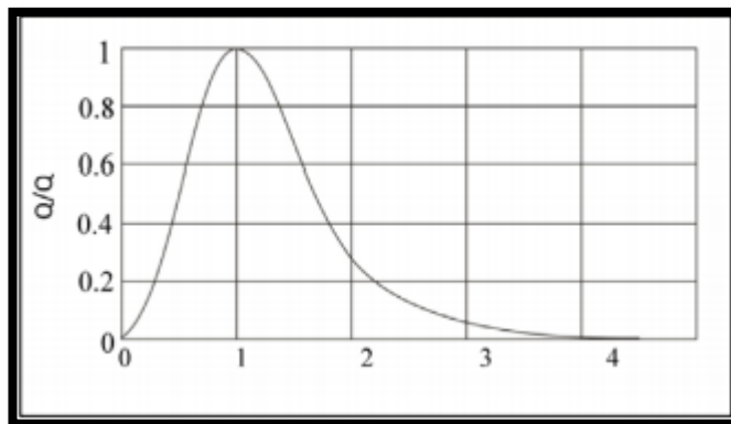
Figura 3. Hidrograma unitario adimensional del SCS. 11
