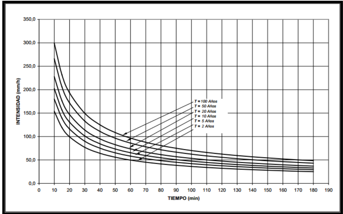
Figura 6. Curvas IDF típicas 20
