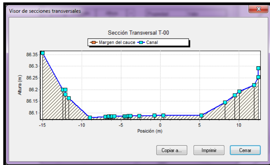
Figura 46. Sección transversal representada en SWMM
