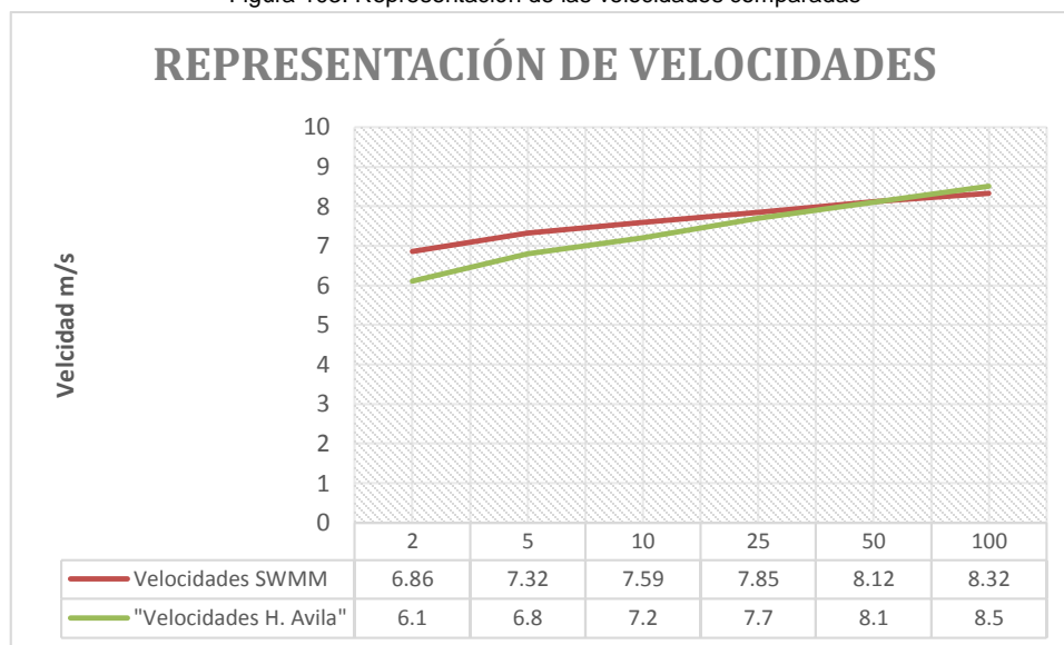
Figura 103. Representación de las velocidades comparadas
