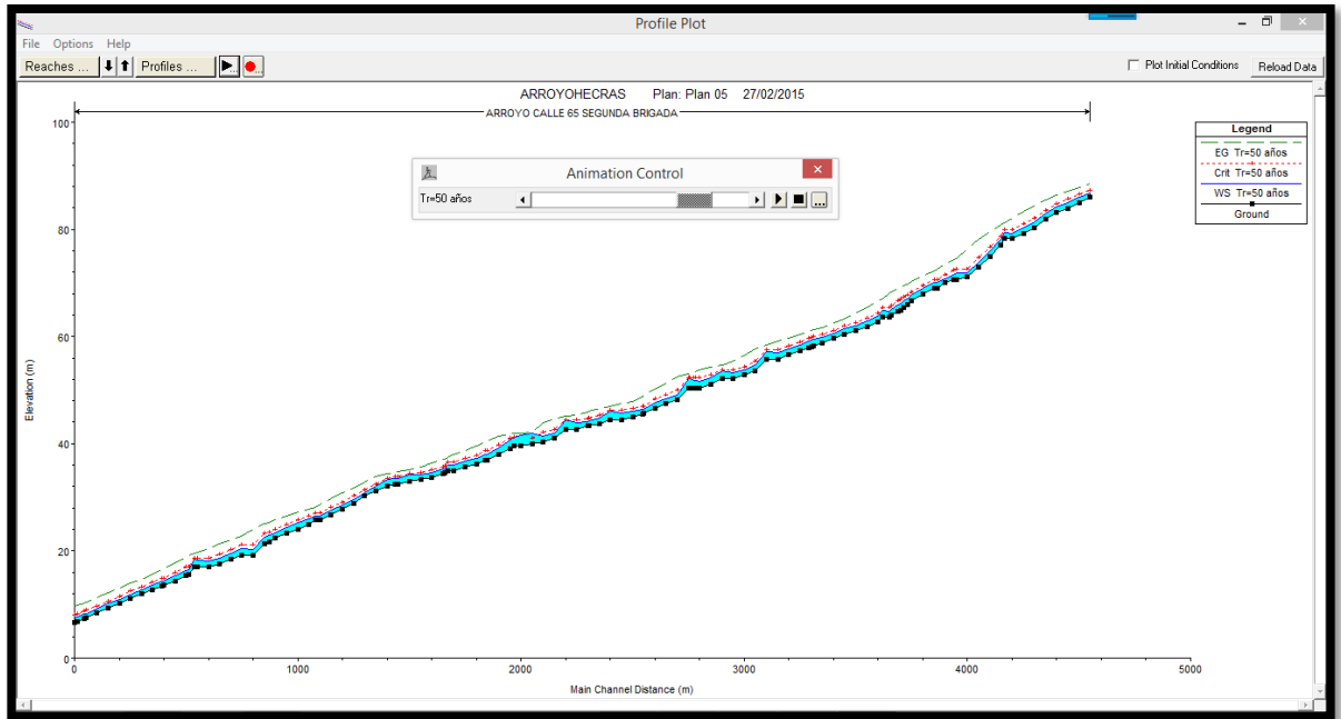
Figura 86. Perfil del arroyo con línea de energía y línea de tirante crítica para un Tr=50 años
